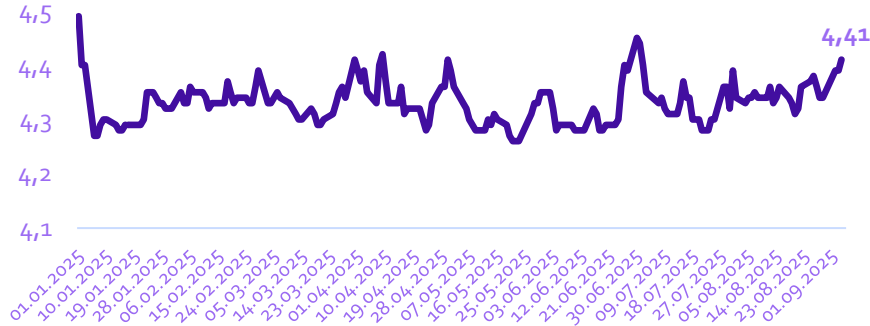
Динамика SOFR
