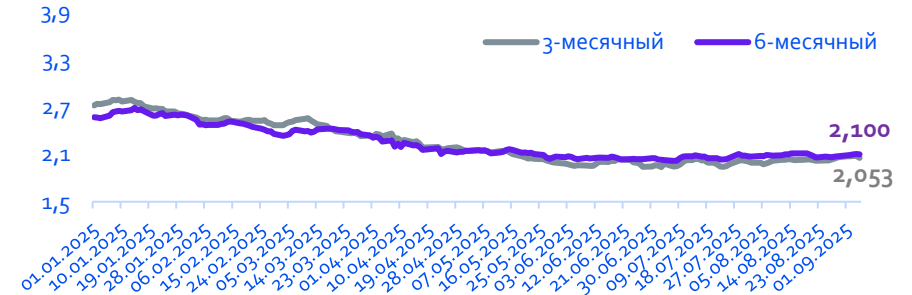
Динамика Euribor
